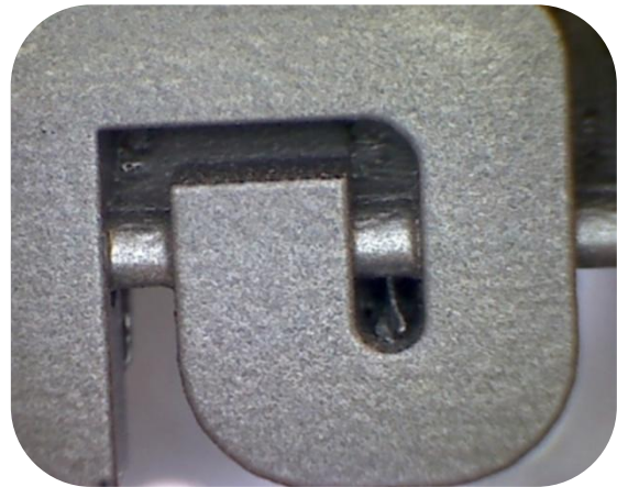
Stahlbauteil-3D Druck
