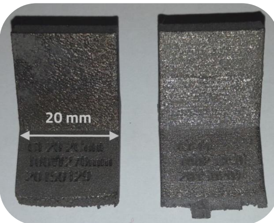
Stahlbauteile-3D Druck
